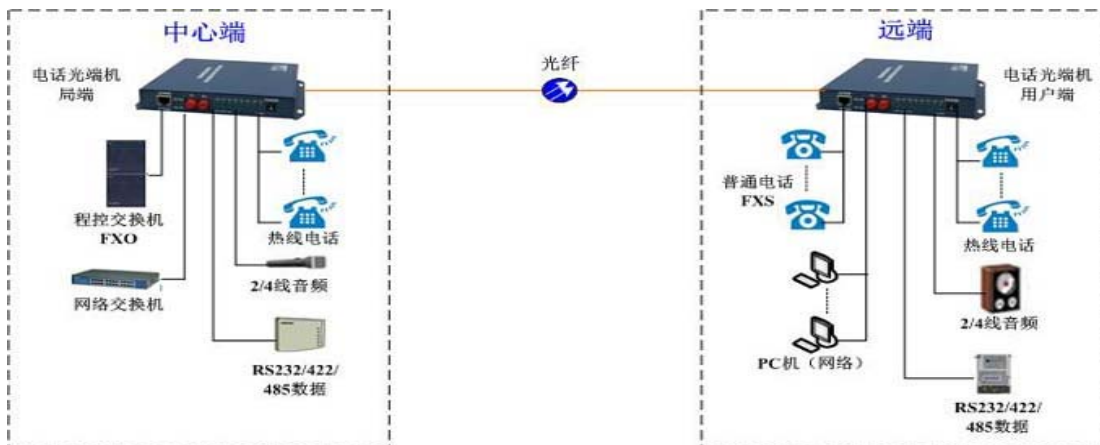
方案一：光纤点对点组网
