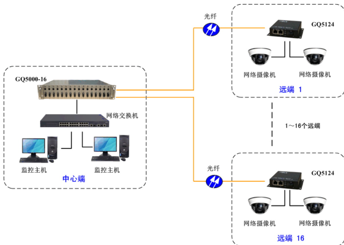
方案二：光纤点对多点组网
